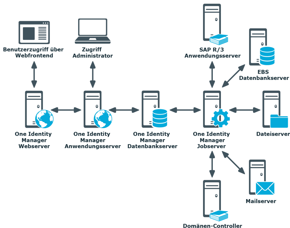
Abbildung 1: Überblick über die One Identity Manager-Komponenten
