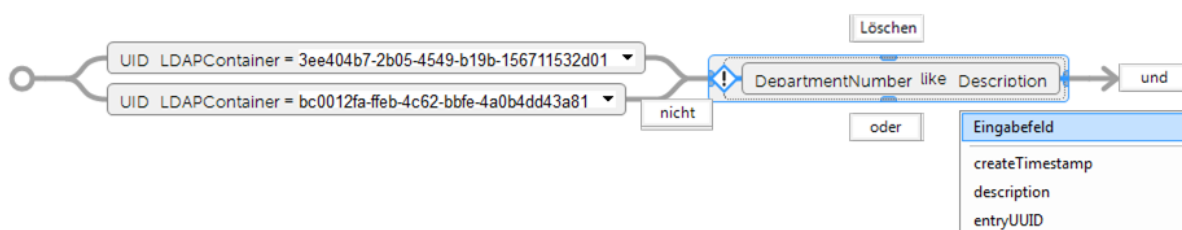
Abbildung 18: Assistent zur Eingabe von Filtern
