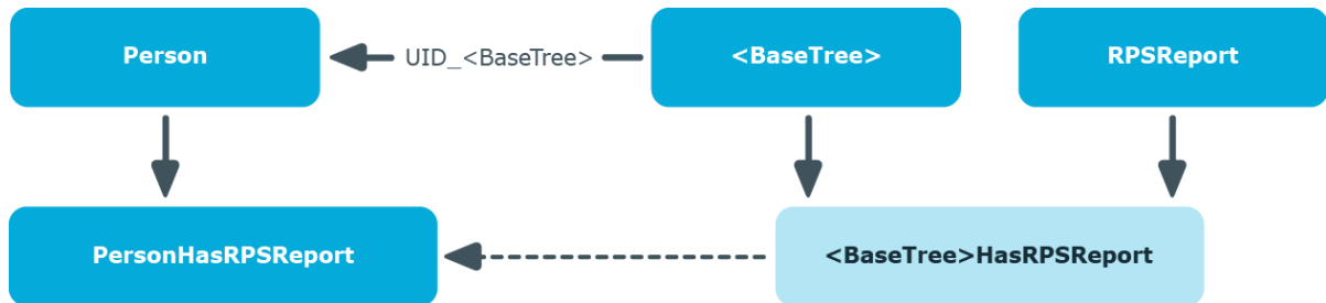
Abbildung 6: Vererbung bei indirekter primärer Zuweisung von abonierbaren Berichten an Identitäten
