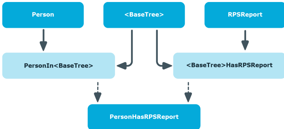
Abbildung 5: Vererbung bei indirekter sekundärer Zuweisung von abonierbaren Berichten an Identitäten
