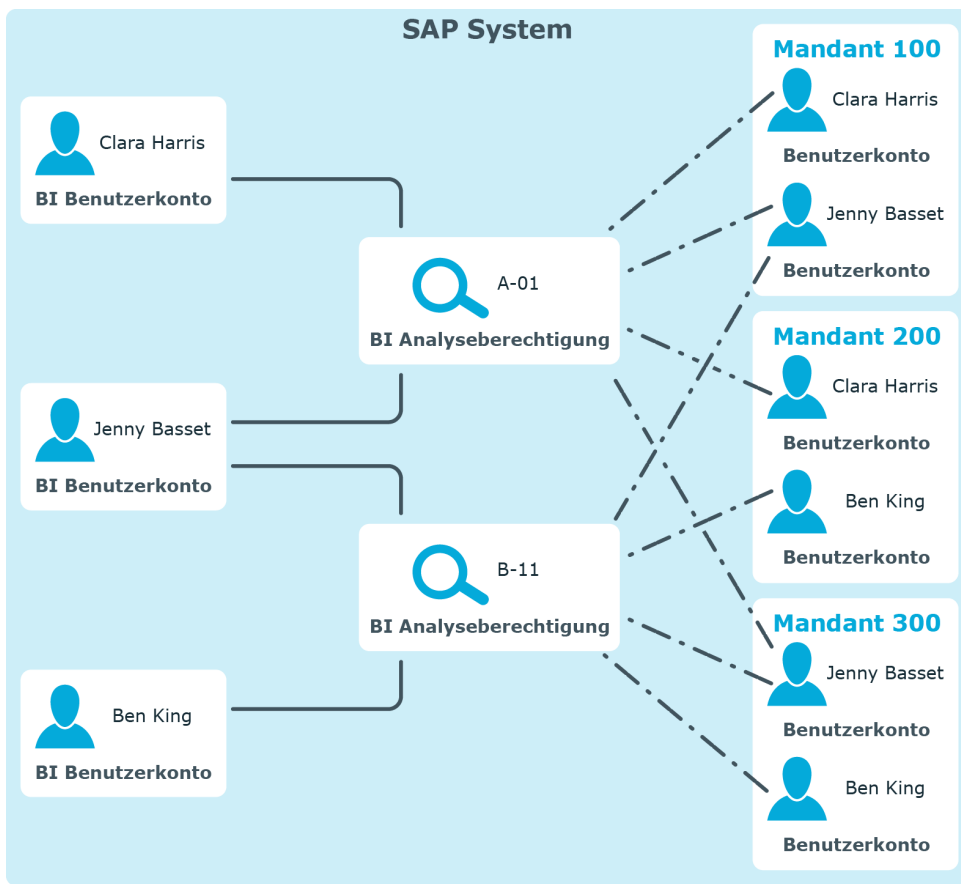
Abbildung 1: Abbildung von BI Analyseberechtigungen im One Identity Manager
