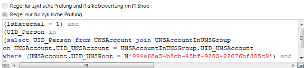
Abbildung 8: Direkte Eingabe der SQL-Abfrage
