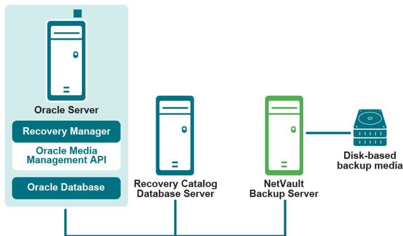
図 3. シングル・インスタンスの非 RAC 設定
