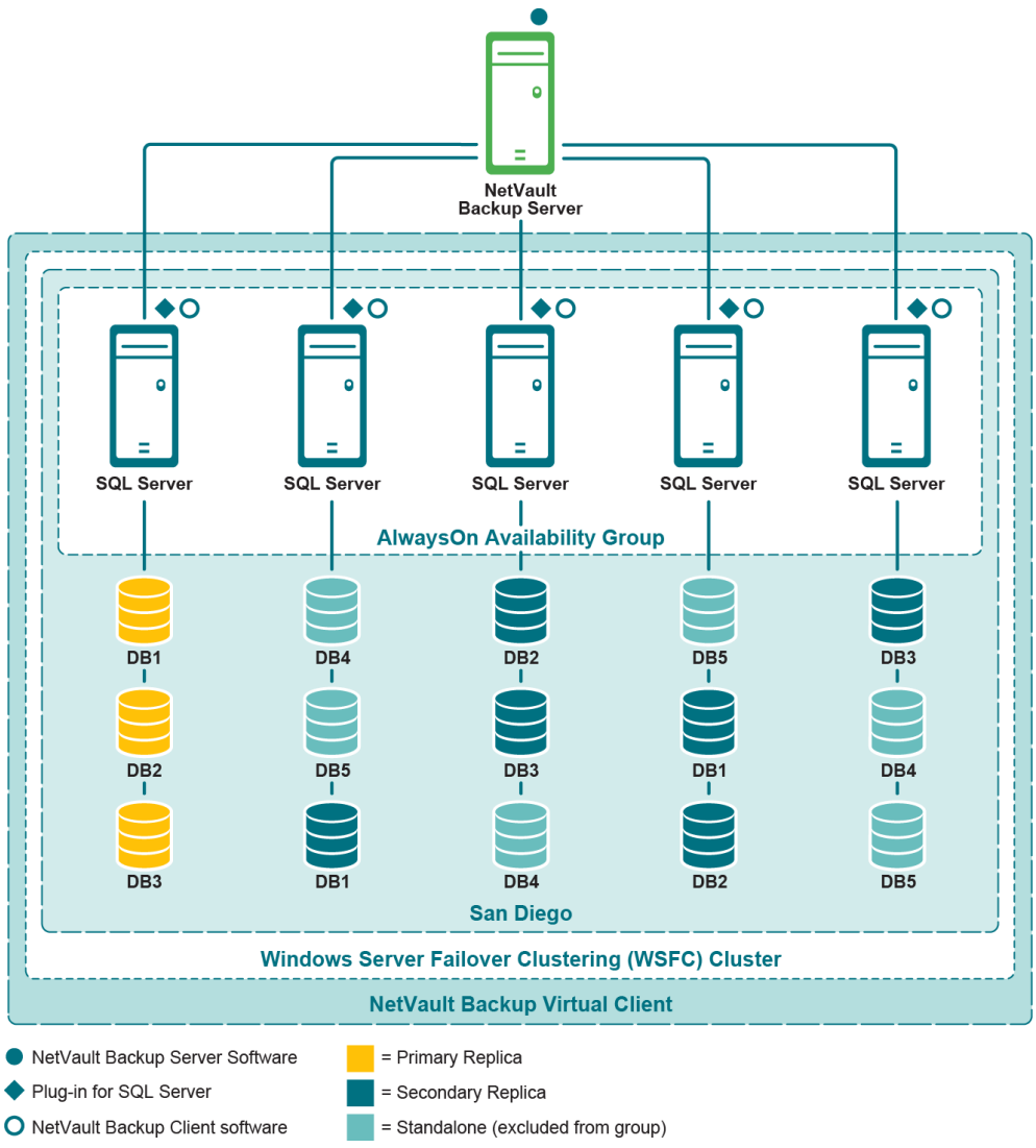
그림 2. AlwaysOn 배포
