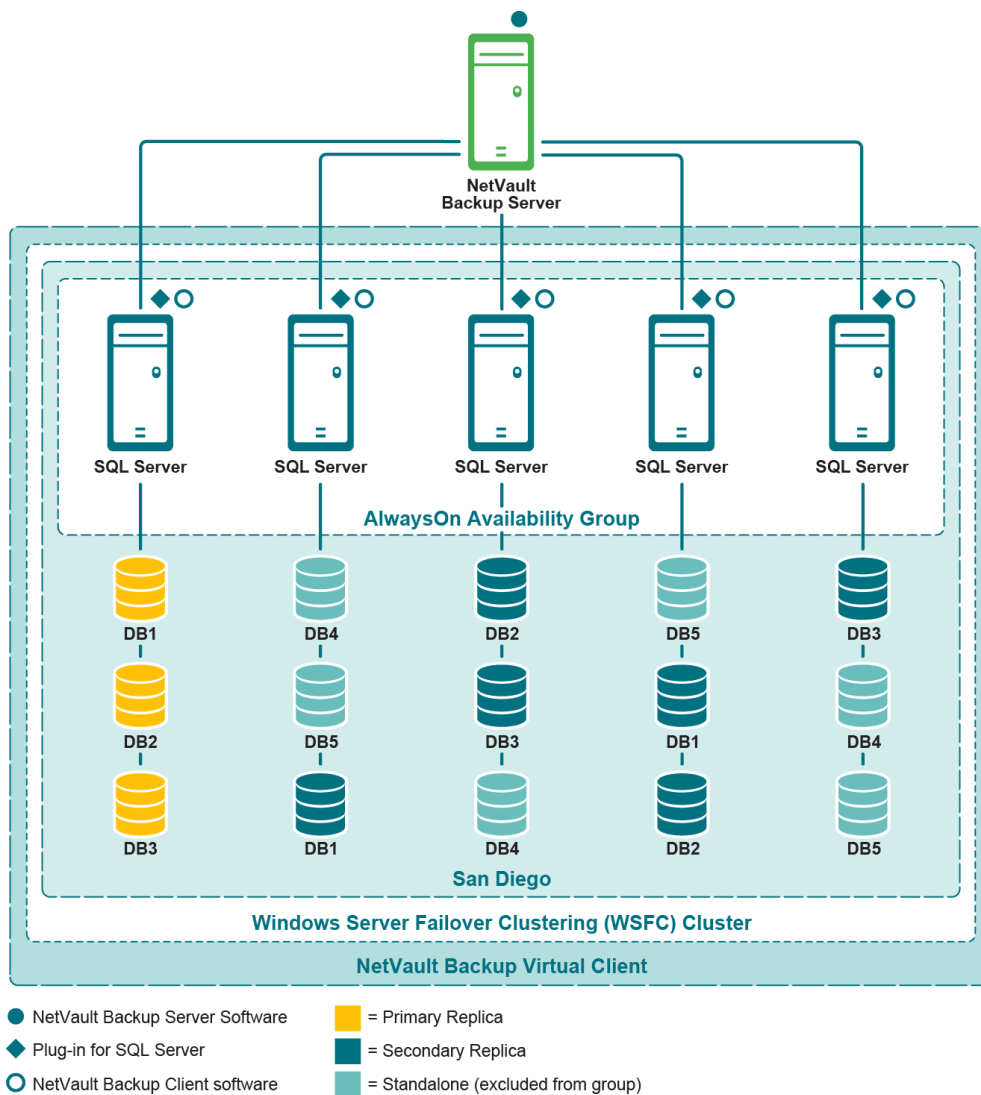
그림 2. AlwaysOn 배포
