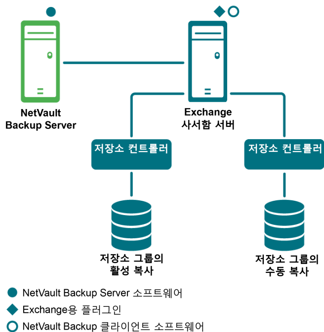
그림 3. LCR 배포
