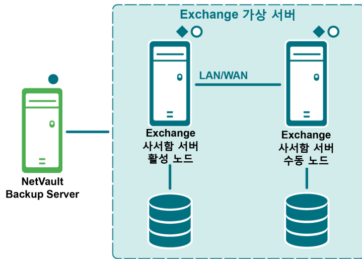
그림 5. CCR 배포
