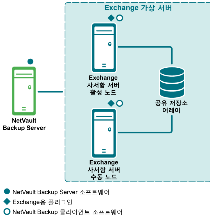
그림 4. SCC 배포
