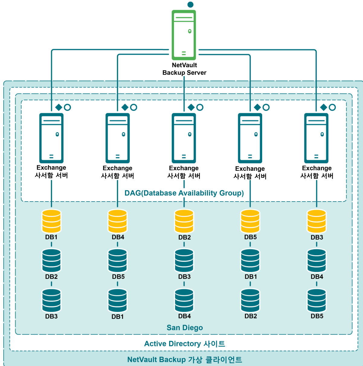
그림 2. DAG 배포
