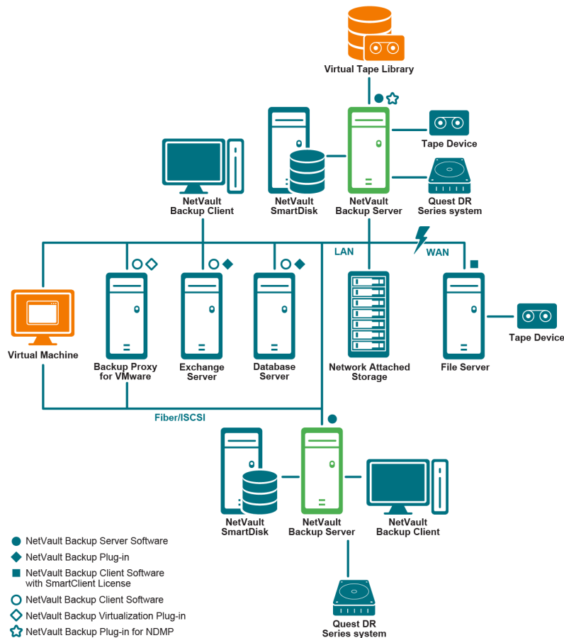
그림 1. NetVault Backup 배포 개요
