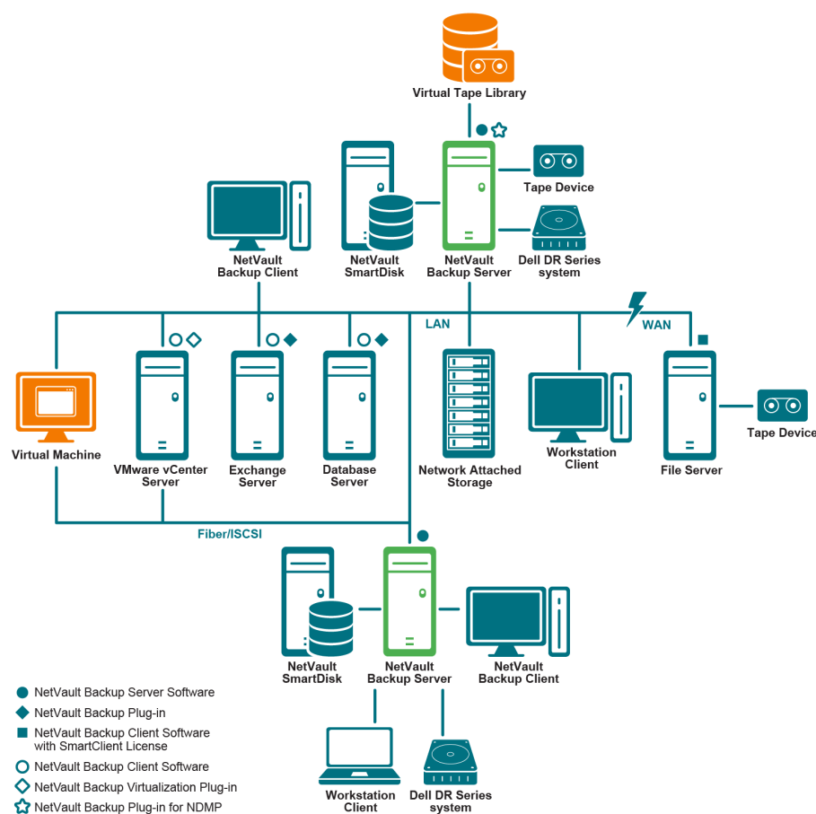
図 1. NetVault Backup 配備の概要
