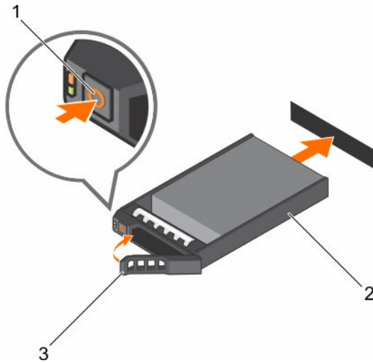
Figure 70. Installation d'un disque dur ou SSD remplaçable à chaud
