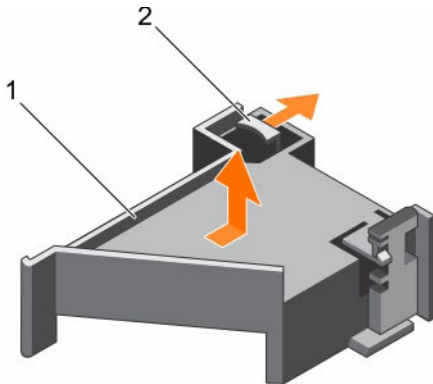
Figure 25. Retrait du support de carte PCIe
