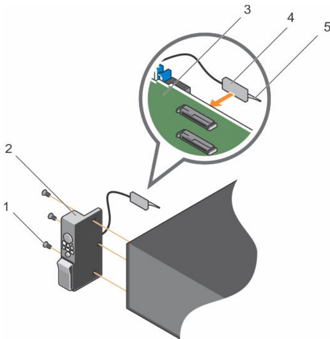
Figure 83. Installation du panneau de commande
