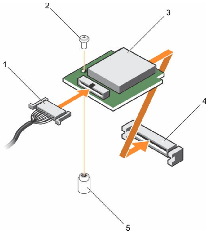
Figure 81. Installation de l'unité de support vFlash
