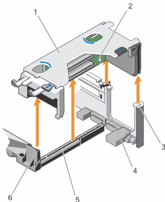
Figure 39. Retrait de la carte de montage pour carte d'extension 1
