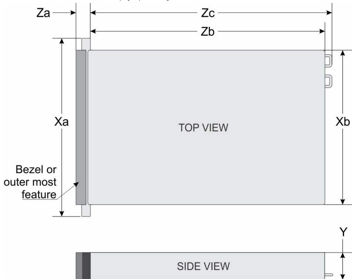
Figure 8. Dimensions du châssis de votre système Dell DR4300
