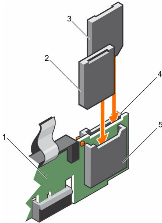
Figure 50. Installation d'une carte SD interne
