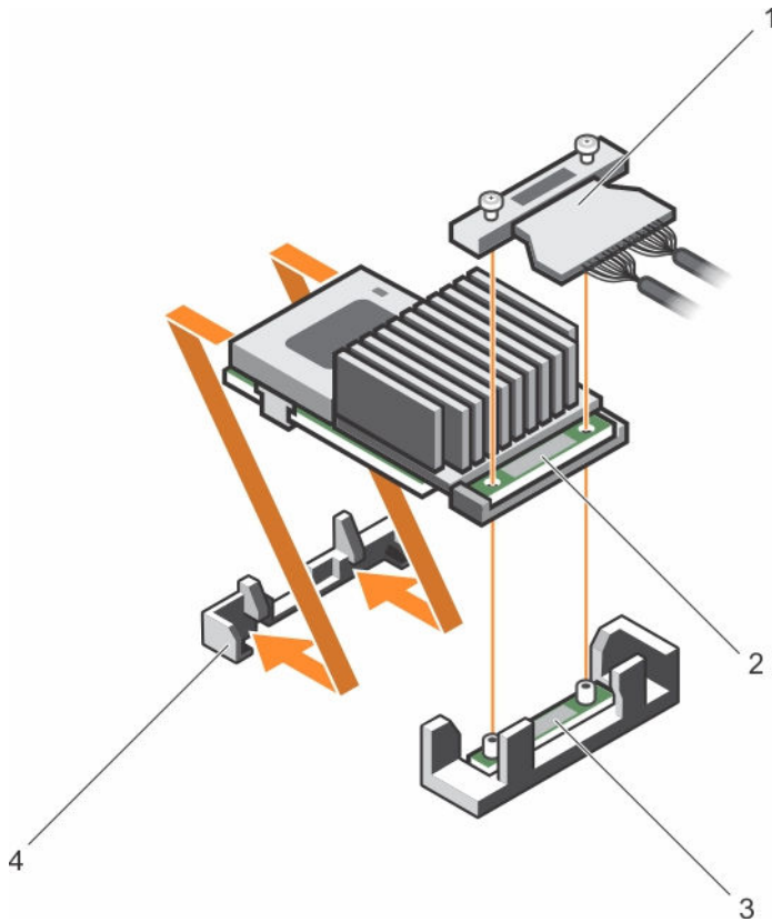
Figure 32. Installation de la carte contrôleur de stockage intégrée
