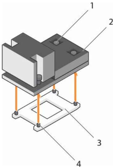
Figure 20. Retrait d'un dissipateur de chaleur
