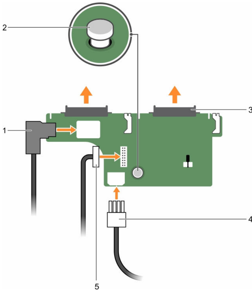
Figure 77. Installation du fond de panier de disque dur (x2) de 2,5 pouces facultatif
