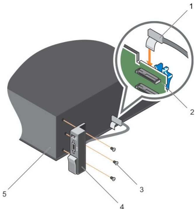
Figure 85. Installation du panneau des entrées/sorties
