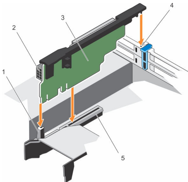
Figure 48. Installation de la carte de montage pour carte d'extension 3
