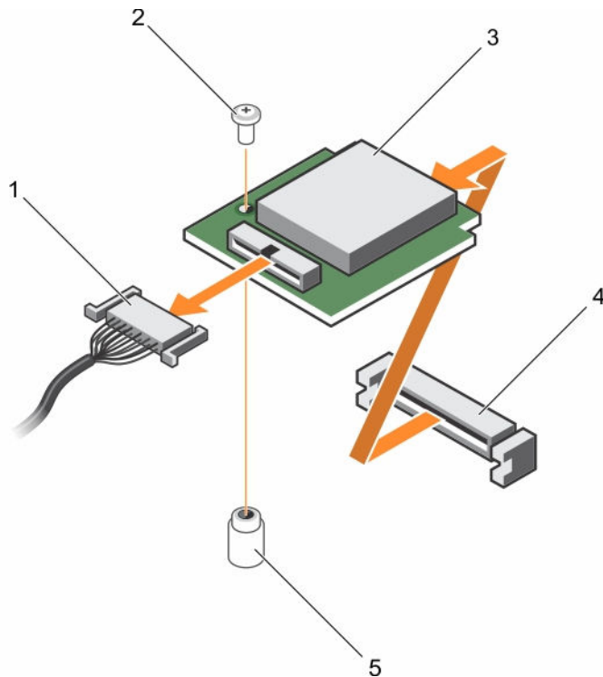
Figure 80. Retrait de l'unité de support vFlash
