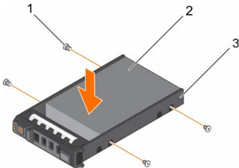
Figure 72. Installation d'un disque dur dans un support de disque dur
