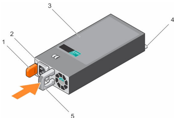
Figure 61. Installation d'un bloc d'alimentation (PSU) CA
