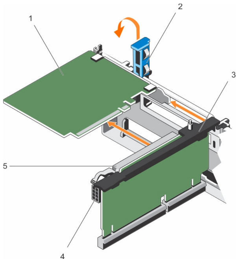
Figure 33. Retrait d'une carte d'extension dans la carte de montage pour cartes d'extension 2 ou 3
