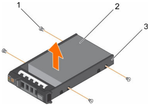
Figure 71. Retrait d'un disque dur d'un support de disque dur
