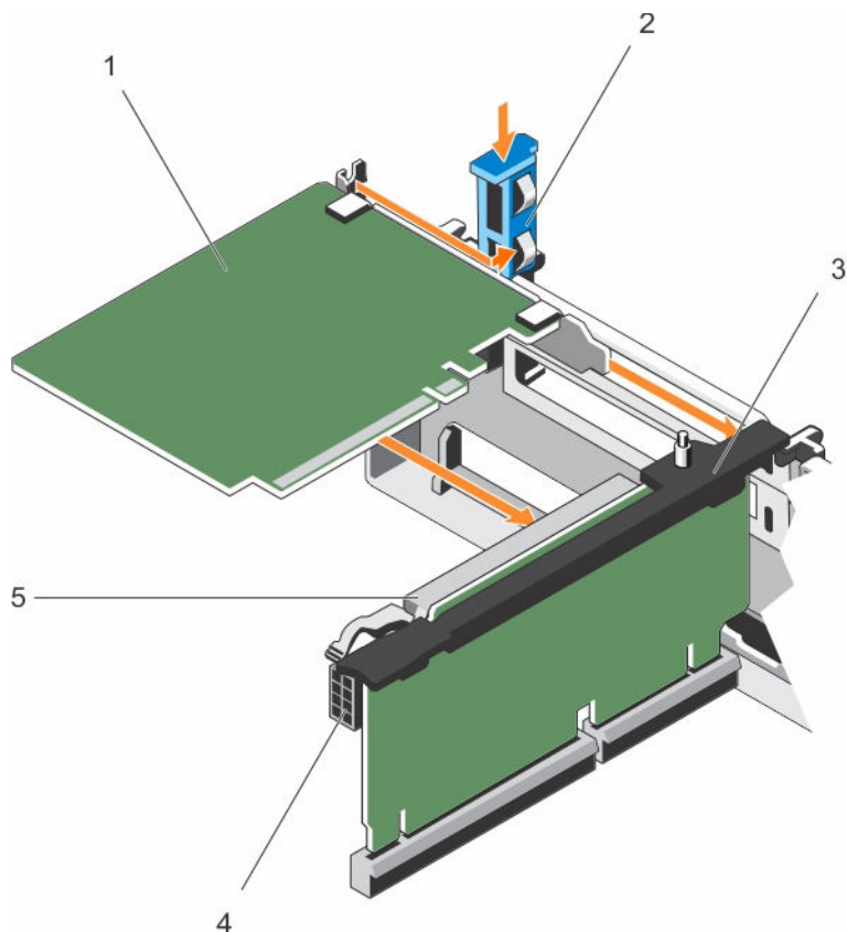
Figure 34. Installation d'une carte d'extension dans la carte de montage pour carte d'extension 2 ou 3
