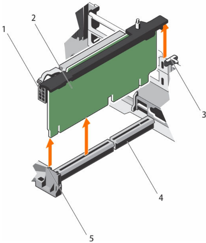
Figure 41. Retrait de la carte de montage pour carte d'extension 2
