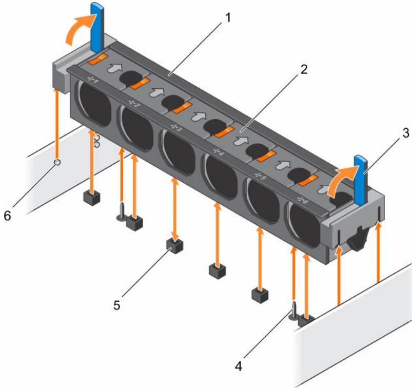
Figure 15. Retrait de l'assemblage de ventilation
