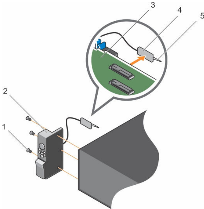
Figure 82. Retrait du panneau de commande
