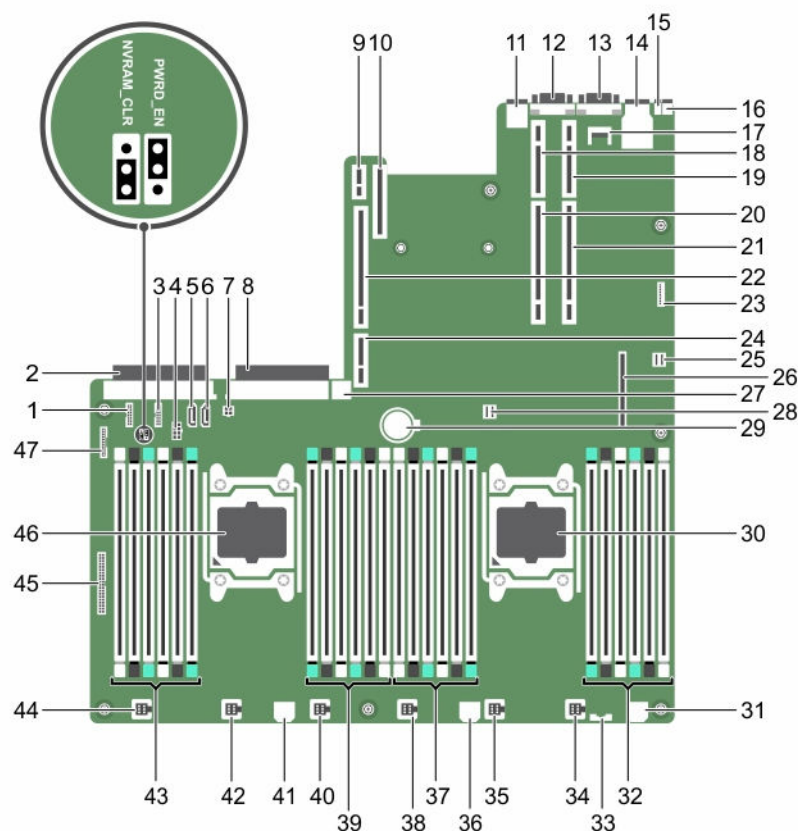
Figure 86. Connecteurs et cavaliers de la carte système
