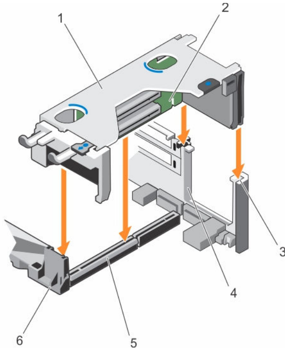
Figure 46. Installation de la carte de montage pour carte d'extension 1
