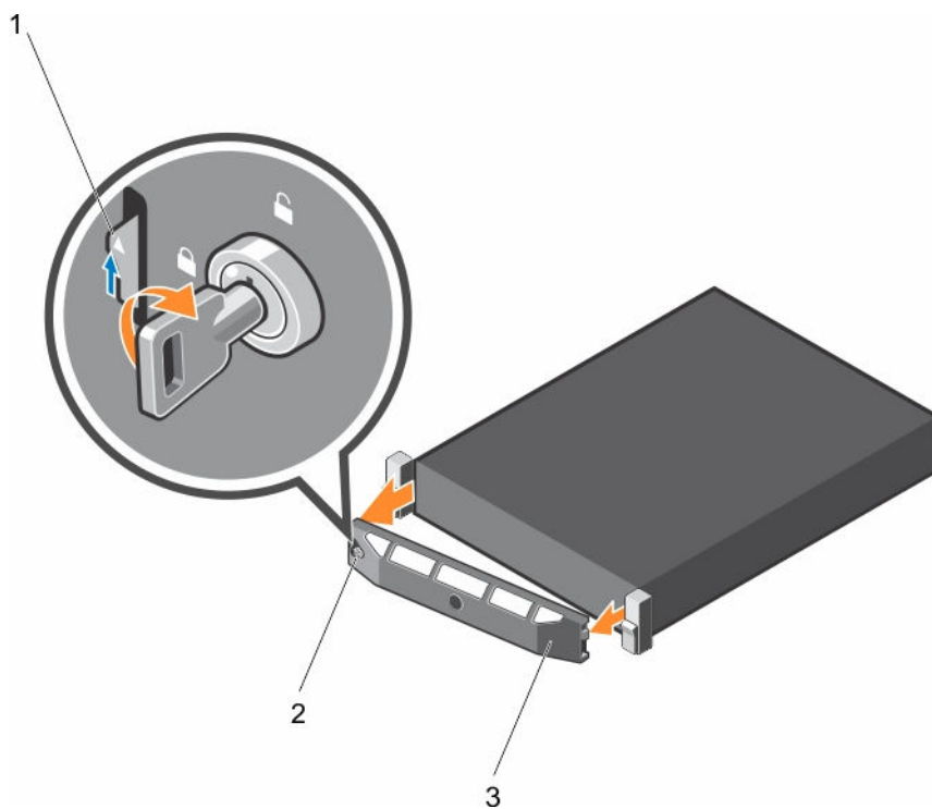
Figure 9. Retrait du cadre avant en option.
