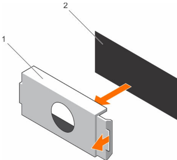
Figure 58. Retrait du cache de PSU
