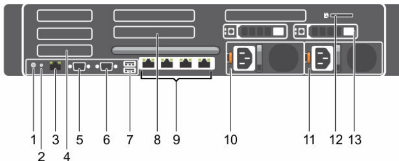
Figure 2. Caractéristiques du panneau arrière
