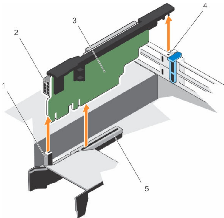
Figure 43. Retrait de la carte de montage pour carte d'extension 3
