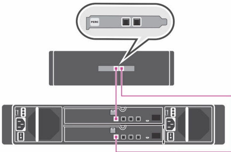
图 2: 将 DL4300 系统连接至 MD1400 存储柜
