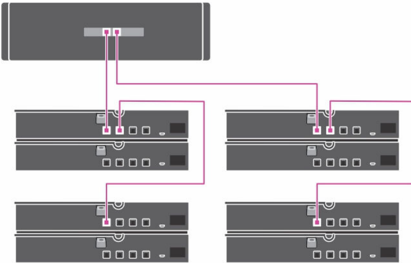
图 3: 多链配置
