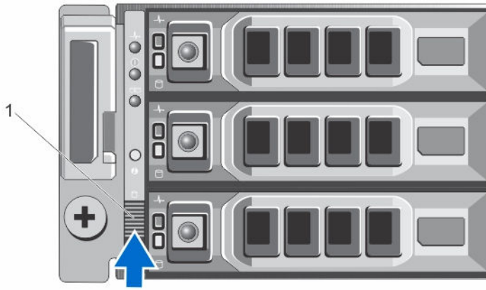
图 1: 设置 PowerVault MD1400 存储柜配置开关
