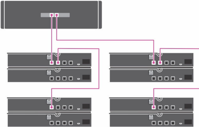
Abbildung 3. Multichain-Konfiguration
