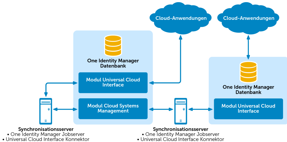
Abbildung 1: Architektur für die Synchronisation
